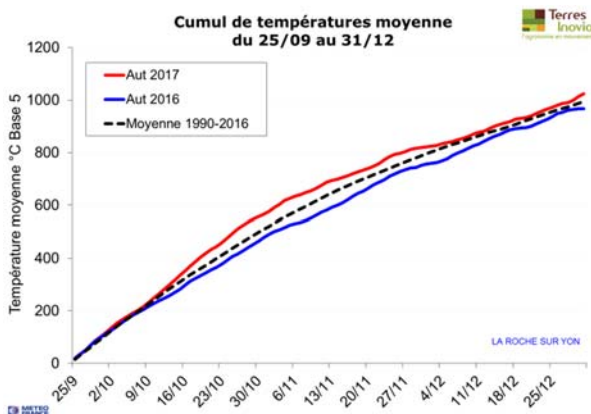
Figure 1 : Cumul de températures base 0 - Automne 2017 station météo de La Roche sur Yon (85)
